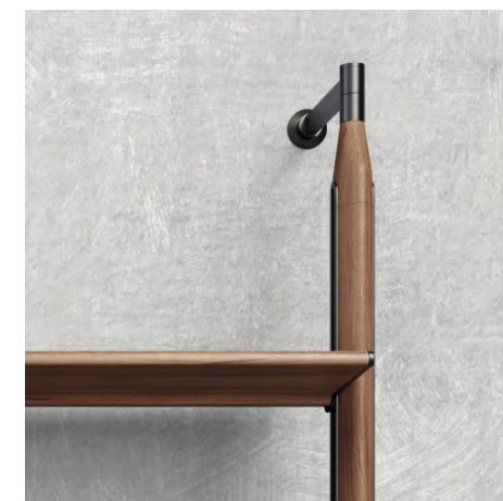
Крепление стойки к стене
