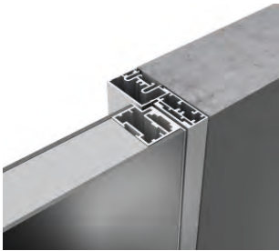
короб MAXI
