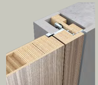
Облицовка откоса гипсокартоном
