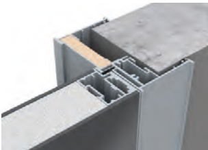
короб PLANAR
